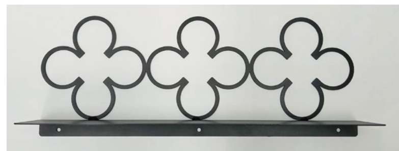
品番 SH-F1 ウォールシェルフ クローバー W500 D100 H191mm
