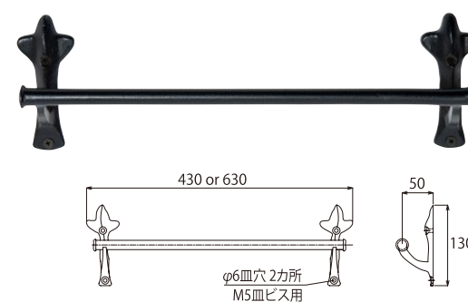
品番 TH-3 タオルハンガー リーフ W430 黒
