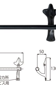
品番 TH-4 タオルハンガー リーフ W630 黒
