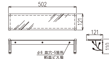
品番 SE-1-W 化粧棚 白 ※ガラスも含む
