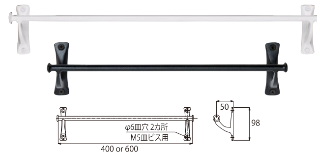
品番 TH-1 タオルハンガー シンプル W400 黒
