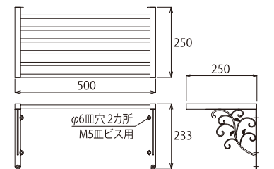
品番 TT-1 タオル棚 黒
