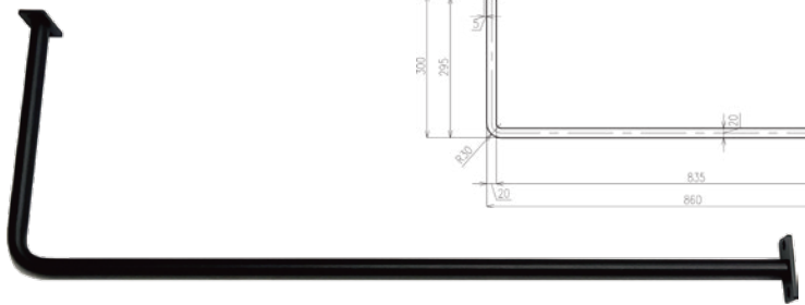
品番 HP3-L850 ハンガーパイプ300 L型850 W865 D70 H300mm
