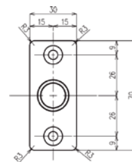
ハンガーパイプ300 取付部 共通サイズ
