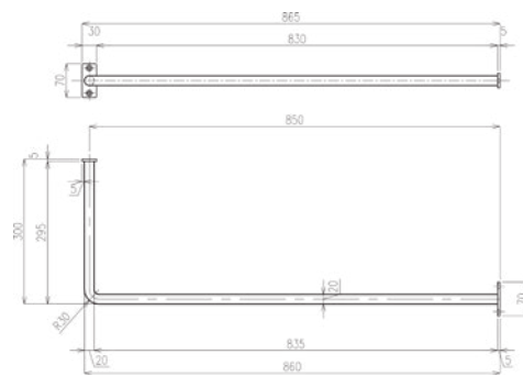
ハンガーパイプ300 取付部 共通サイズ
